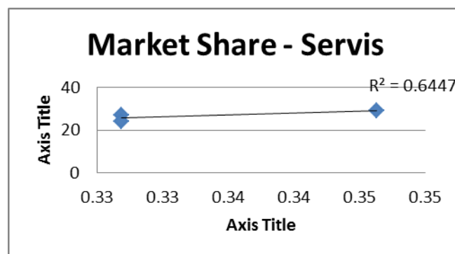
Gambar 3. Grafik Perhitungan R2 Faktor Service dengan Market Share
