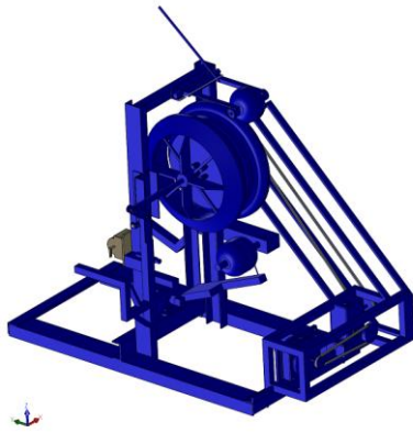
Gambar 3 Desain Mesin Pembuat Marset
