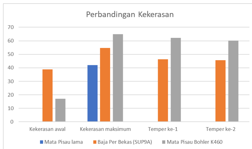
Gambar 8. Grafik Perbandingan Angka Kekerasan
